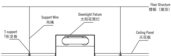
Section Description 安装剖面图
